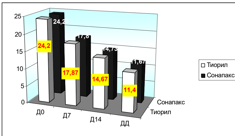
Рисунок 2 – Динамика показателей тревоги по шкале Гамильтона в обследованных группах больных
